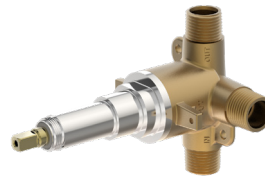
Dual Outlet Diverter Valve Body 2DIVBODYSRT GH-502-06
